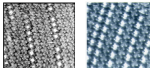
混合ポルフィリン分子膜の配列制御
