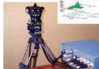
超音波アレイセンサーと位置測定結果
