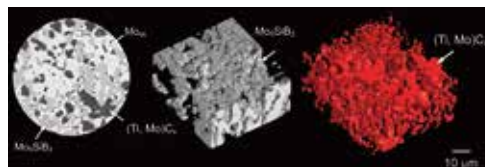
次世代航空機ジェットエンジン用超高温材料として開発が進められているMoSiB 2 C合金を2次元走査型電子顕微鏡像と同視野からMo 5 SiB 2 相のみを抽出した3次元像
