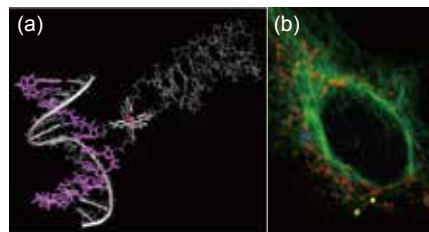
(a) 金属イオンの刺激に応じてダイナミックに構造を変化させる人工核酸 (b) 核酸アプタマーを利用したmRNAグラニュールのライブセルイメージング
