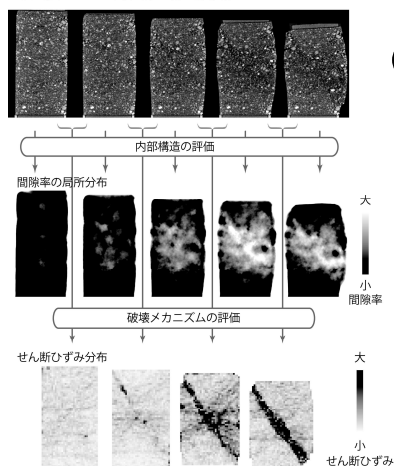
(社基-2) X線CTによる画像解析の一例
