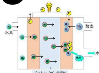
水素型燃料電池の作動メカニズム
