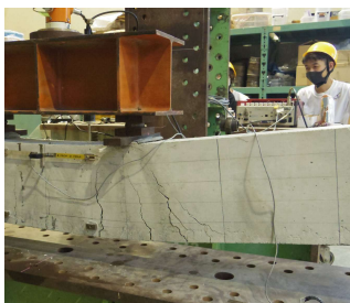
鉄筋コンクリート梁の曲げ載荷実験 構造部材である鉄筋コンクリート梁の強さを曲げ載荷実験により調べています。
