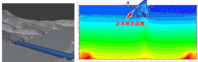
（社基-3）ダムの設計・数値シミュレーション
