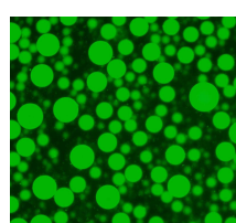
液液相分離で形成される液滴
